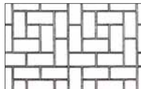
középtéglás kötés
